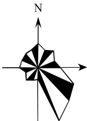
图 2 16 方向风向玫瑰图（示例）
